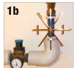
senkrechte Montage
